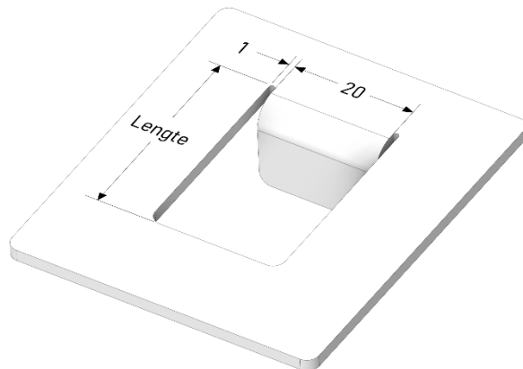
Ingesloten zetting
